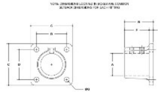
#45CE Square Base Flange SCALE: 1:1
