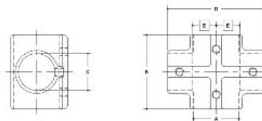
#7-89 Cross SCALE: HALF
