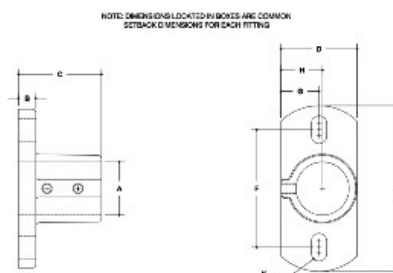
#46 Base Flange SCALE: 1/4"=1"
