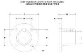
M42 Round Base Flange DIN 934, 934P
